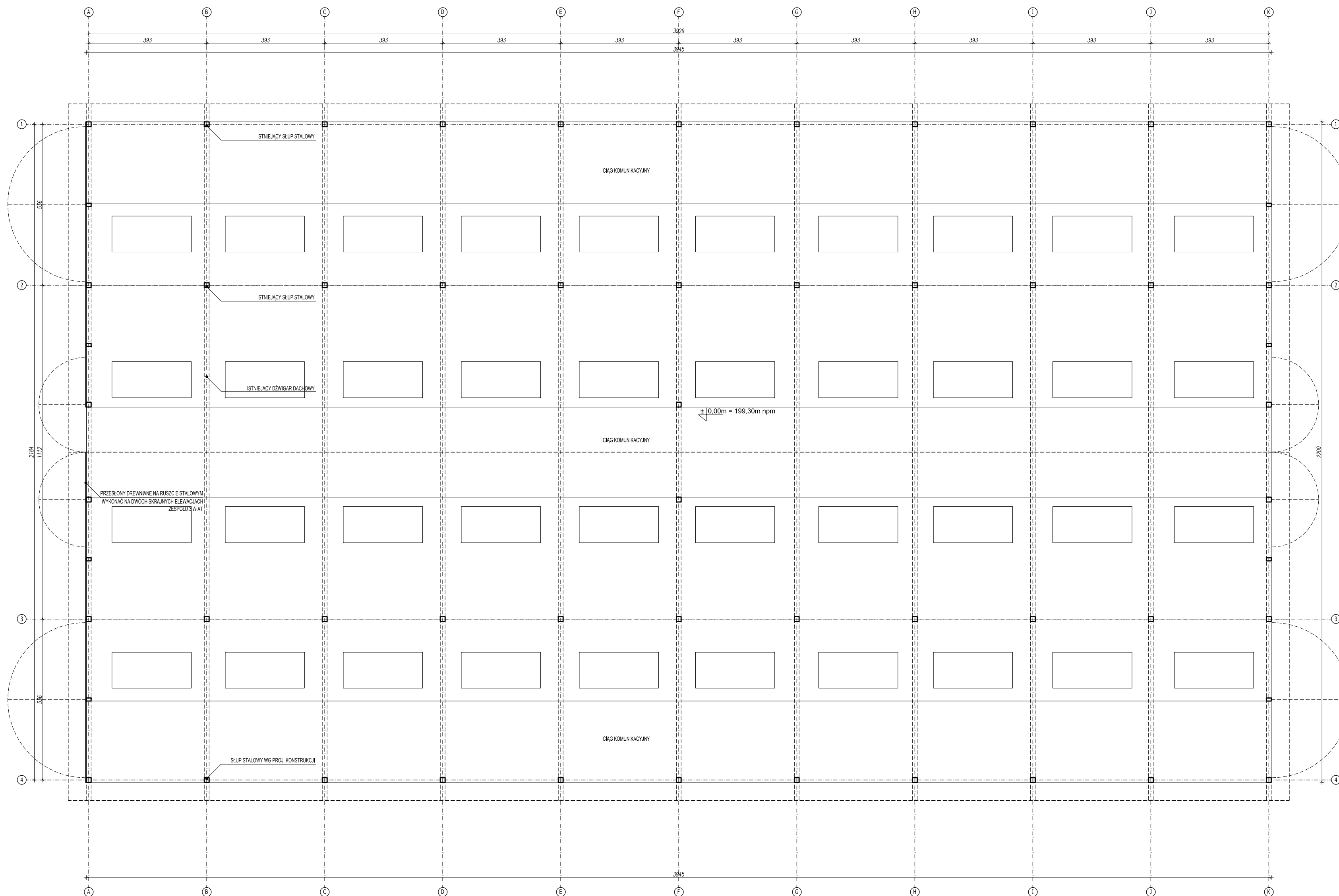
RZUT PRZYZIEMIA SKALA 1:100
